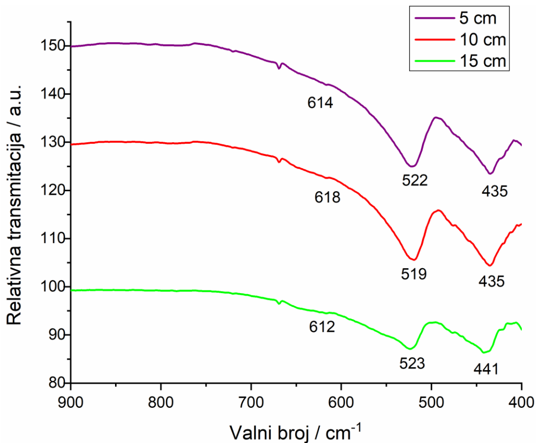
Slika 4.2. ATR-FTIR spektri elektroispredenih vlakana sintetiziranih pri različitim udaljenostima; 5 cm, 10 cm i 15 cm te istoj brzini protoka 1,0 \text{ mL h}^{-1} i naponu od 10 kV. Spektri su snimljeni nakon termičke obrade vlakana ( T = 500 \text{ }^{\circ}\text{C} , 4 sata) u području valnih brojeva od 4000 do 400 \text{ cm}^{-1} na T = 22 \pm 2 \text{ }^{\circ}\text{C} . Na slici su prikazani spektri u području od 900 do 400 \text{ cm}^{-1} .
