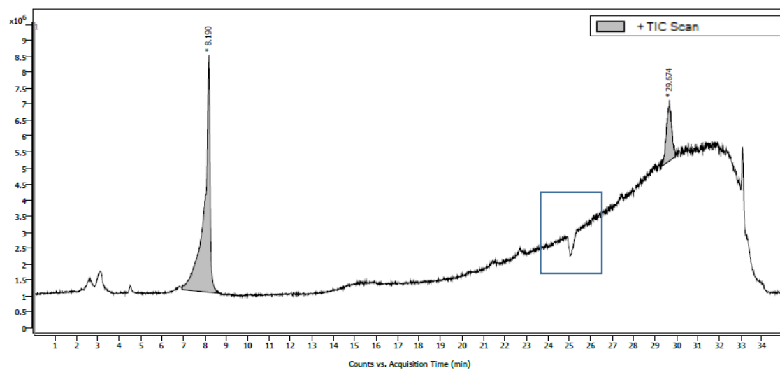
Slika 32. Prikaz pada mase za klozental.
