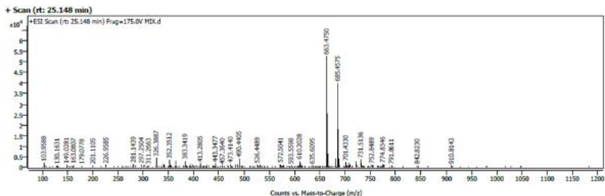
Slika 30. Maseni spektar klotantela.
