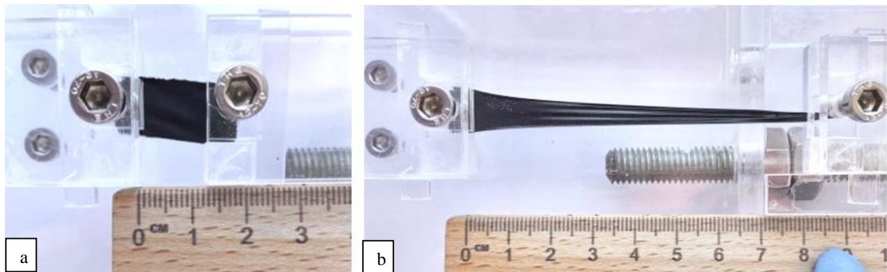
Slika 43. PEDOT-Br:S-SEBS film a) prije istezanja b) pri maksimalnom istezanju
