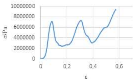
Graf ovisnosti sila - naprezanje za uzorak 4H1
