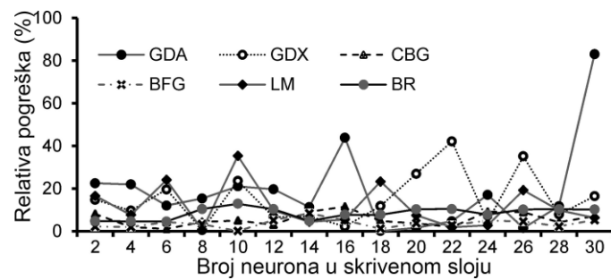
Slika 28. Broj neurona u skrivenom sloju za \text{NO}_x
