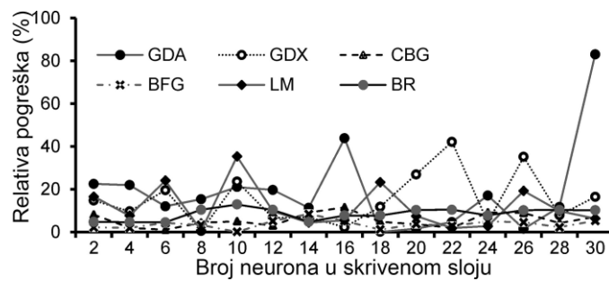
Slika 28. Broj neurona u skrivenom sloju za \text{NO}_x
