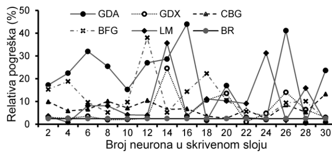
Slika 29. Broj neurona u skrivenom sloju za \text{CO}
