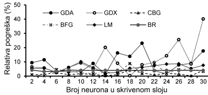
Slika 27. Broj neurona u skrivenom sloju za \text{CO}_2
