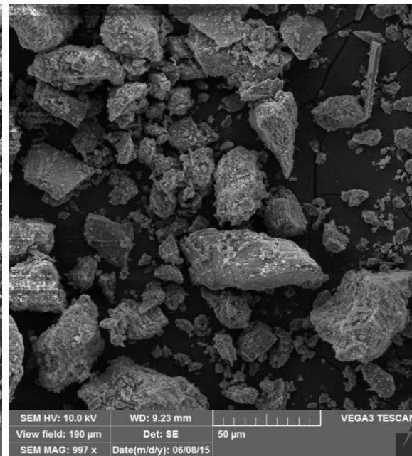
f) Klinoptilolit + DMMP (1000 ×)
