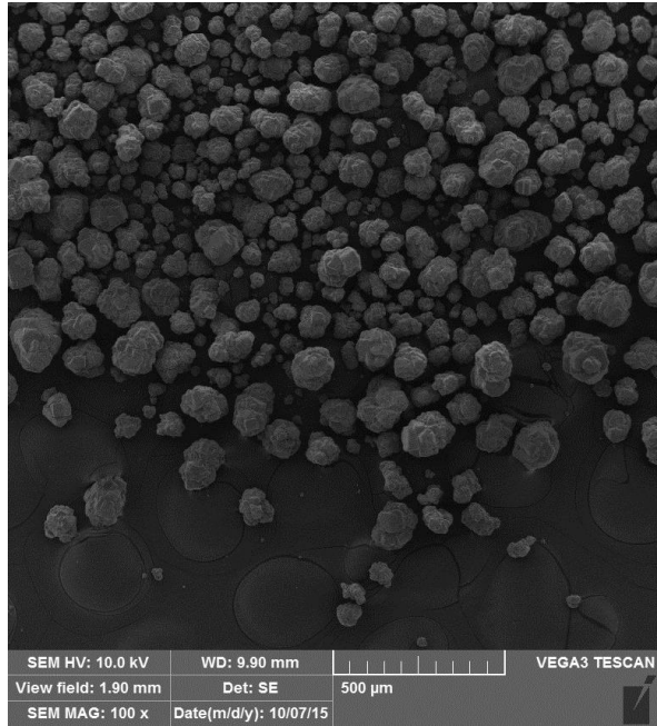
b) \text{Al}_2\text{O}_3 + 2\text{-CEES} (100 ×)
