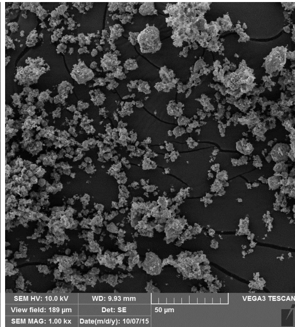
d) Klinoptilolit + MCC Na (1000 ×)
