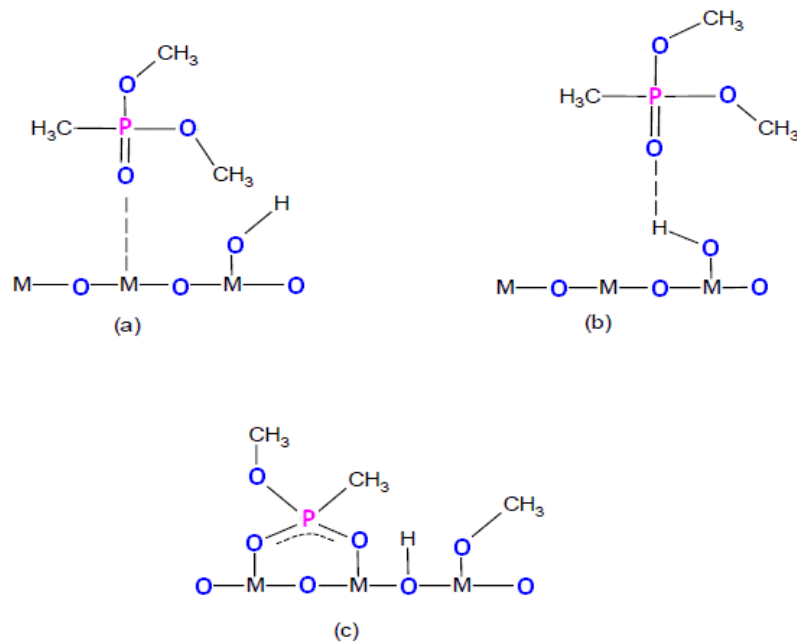
Slika 63. Predložena struktura a) adsorpcije DMMP na Lewis-ovu bazu, b) adsorpcije DMMP na aktivni položaj Brønsted-ove baze (hidroksilna pozicija), c) disocirani DMMP duž površinski vezane metoksi skupine [30]
