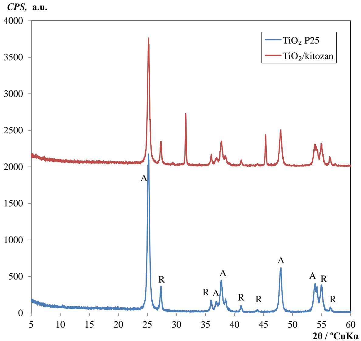
Slika 4.17. Rendgenski difraktogram komercijalnog uzorka \text{TiO}_2 (P25) korištenog za pripremu fotokatalitičkog sloja i \text{TiO}_2 modificiranog kitozanom (A – anatazni oblik, R – rutilni oblik)
