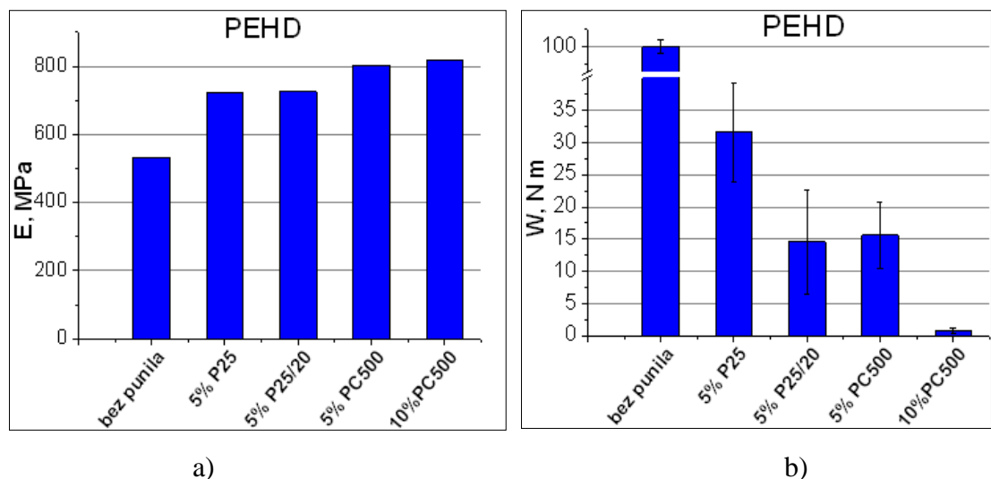
Slika 39: Usporedba mehaničkih svojstava čiste komponente PE-HD i nanokompozita PE-HD: Youngov modul (a); rad loma (b)
