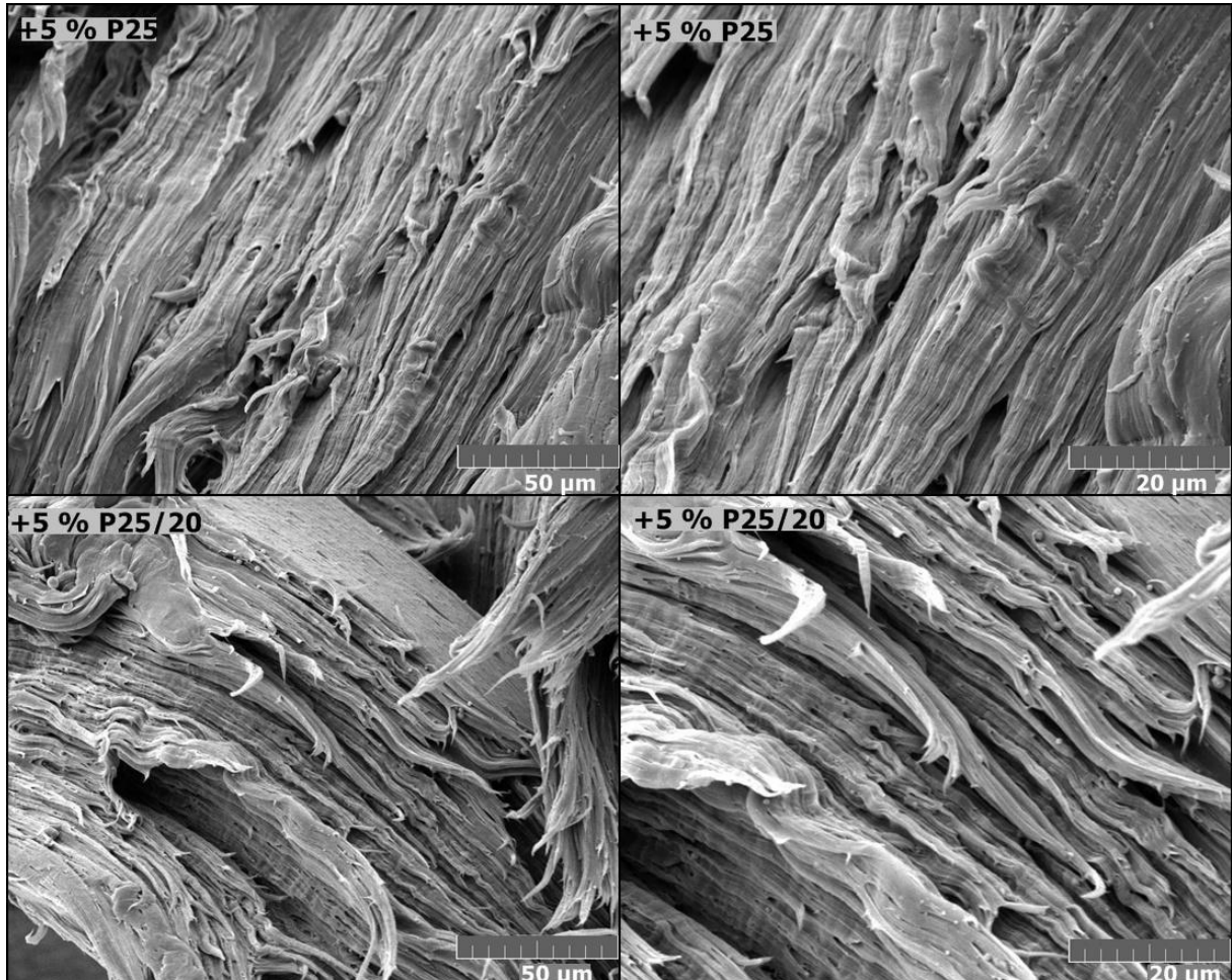
Slika 48: SEM mikrografije površine loma PE-LD s 5 % nanopunila P25 i 5 % nanopunila P25/20
