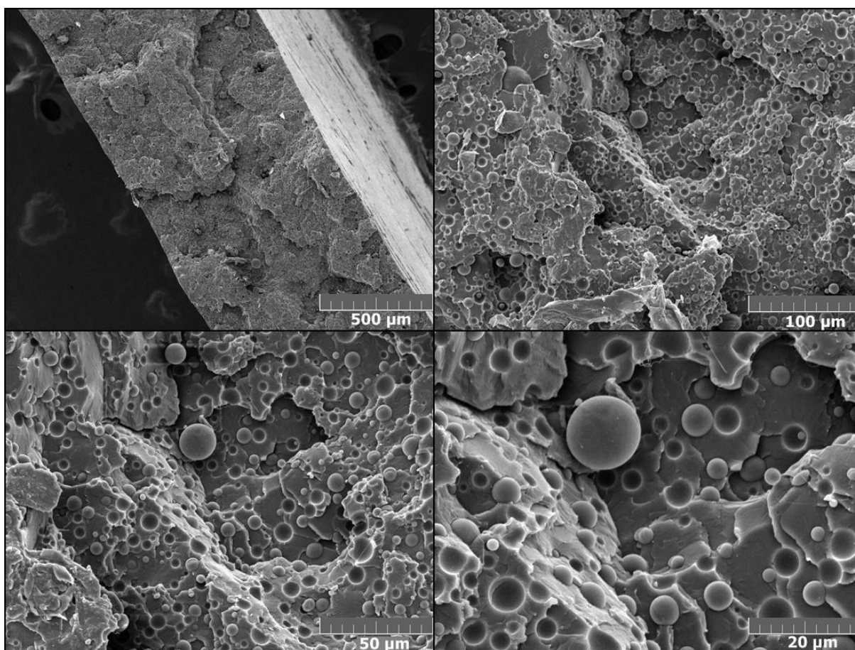
Slika 52: SEM mikrografije površine loma mješavine PLA/PE-HD 90/10 bez punila
