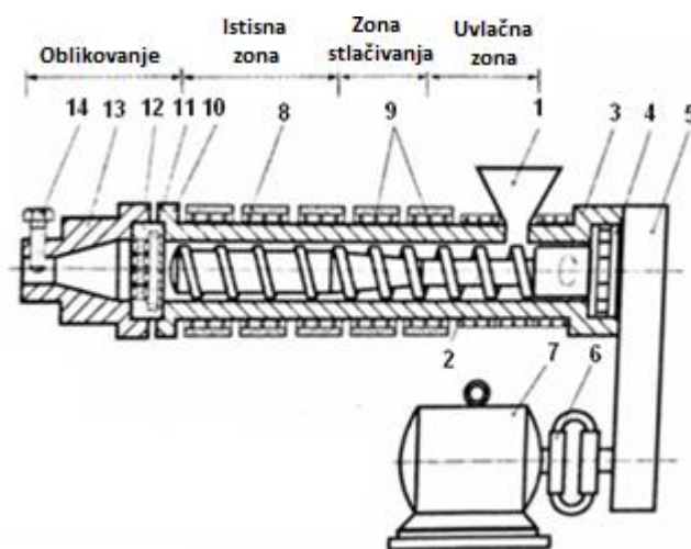
Slika 24: Presjek jednpužnog plastificirajućeg ekstrudera; 1-lijevak, 2-pužni vijak, 3-cilindar, 4-tlačni ležaj, 5-namjestivi prigon, 6-spojka, 7-pogonski motor, 8-grijala, 9-hladila, 10-prirubnica, 11-sita, 12-cjedilo, 13-glava ekstrudera, ujedno i mlaznica, 14-prigušnica ( G.Menges ) 6
