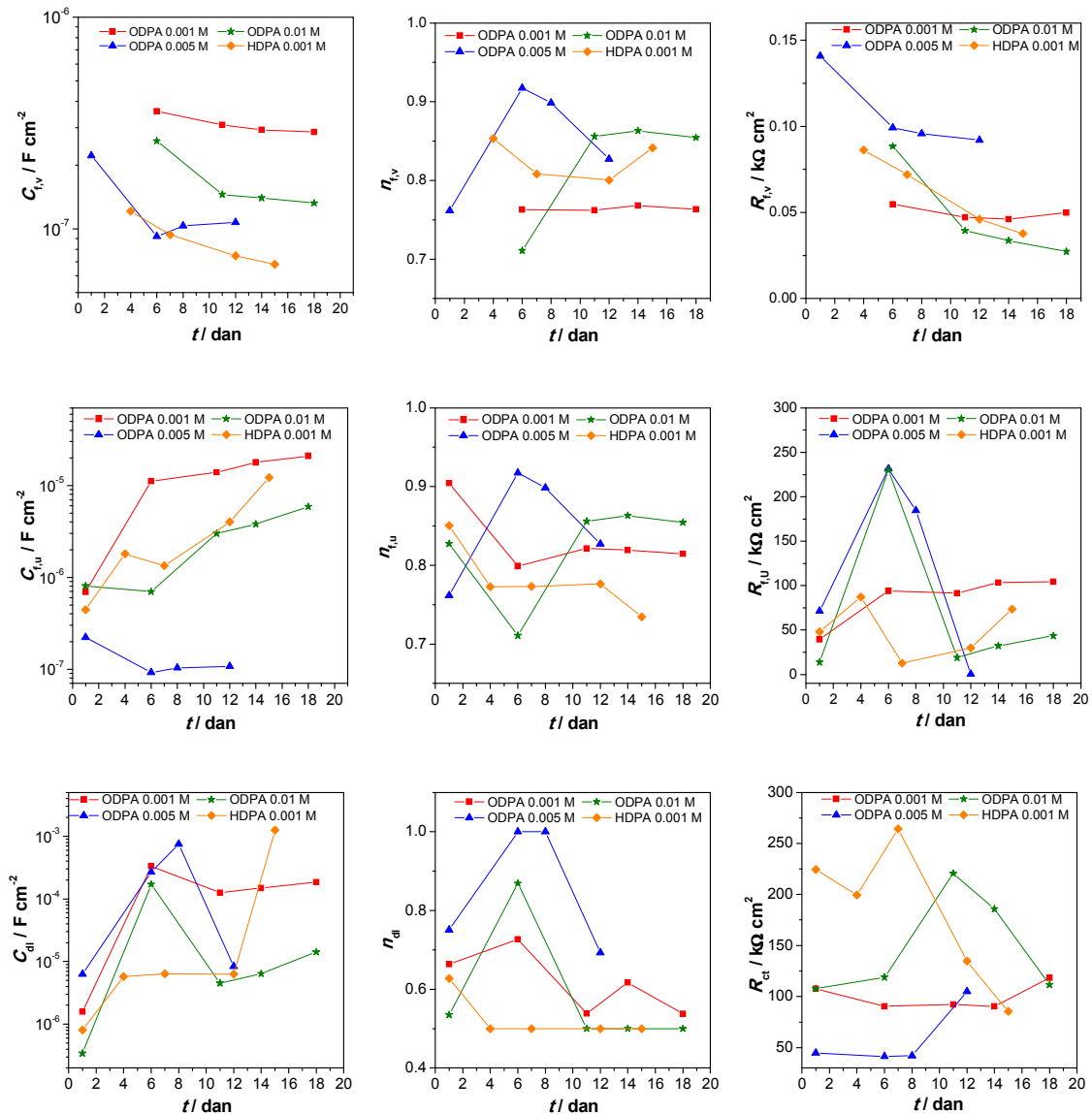
Slika 4.77. Impedancijski parametri dobiveni za sve tri koncentracije ODPa i za 0,001 M HDPa
