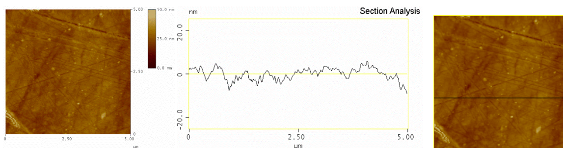
Slika 4.92. AFM slika uzorka tretiranog OK 0,001 M nakon brisanja etanolom
