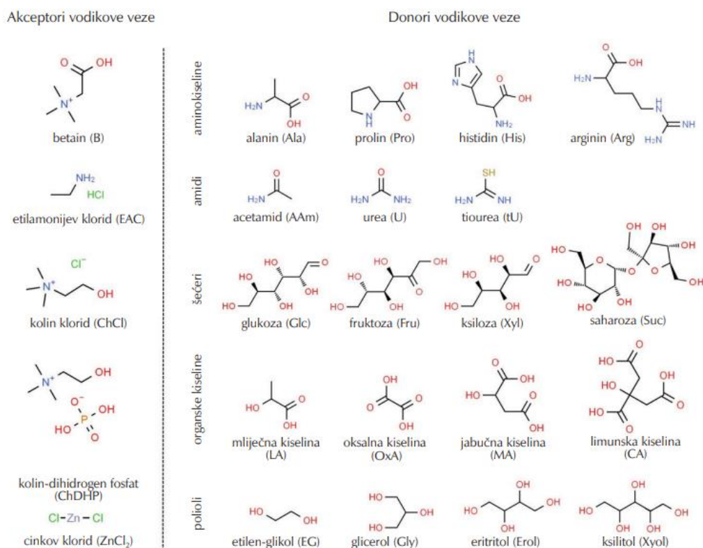
Slika 1. Primjeri spojeva za pripravu niskotemperaturnih eutektičkih otapala 2
