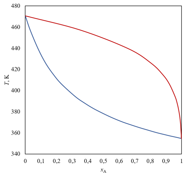
Slika 3. Dijagram vrelišta.
