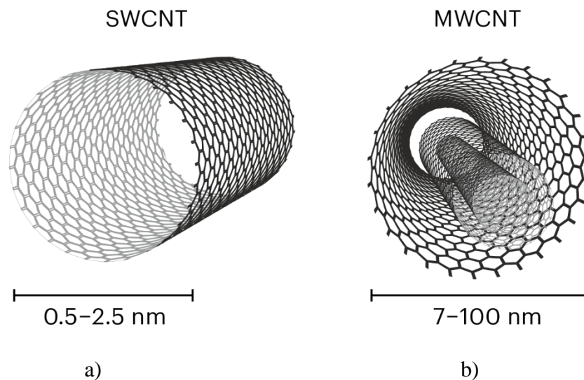
Slika 3. Podjela nanocijevi prema broju slojeva grafena: a) SWNT, b) MWCNT [10]
