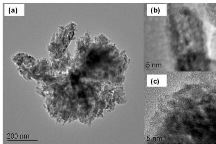
Slika 53. TEM analiza korozijskih produkata s niskom rezolucijom (a) i visokom rezolucijom odabranih područja (b-c), smjesa željeznih hidroksida (npr. \alpha -FeOOH) [31].
