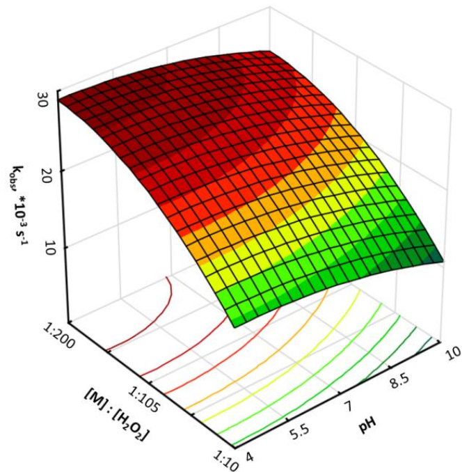
Slika 35. 3D dijagram utjecaja pH vrijednosti i koncentracije H_2O_2 na brzinu razgradnje modelne otopine klorfenvinfosu.
