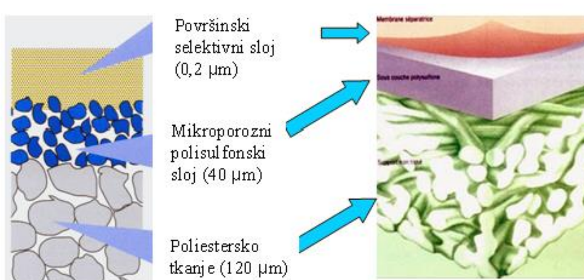
Slika 2.2. Presjek tankoslojne kompozitne membrane (TFC).
