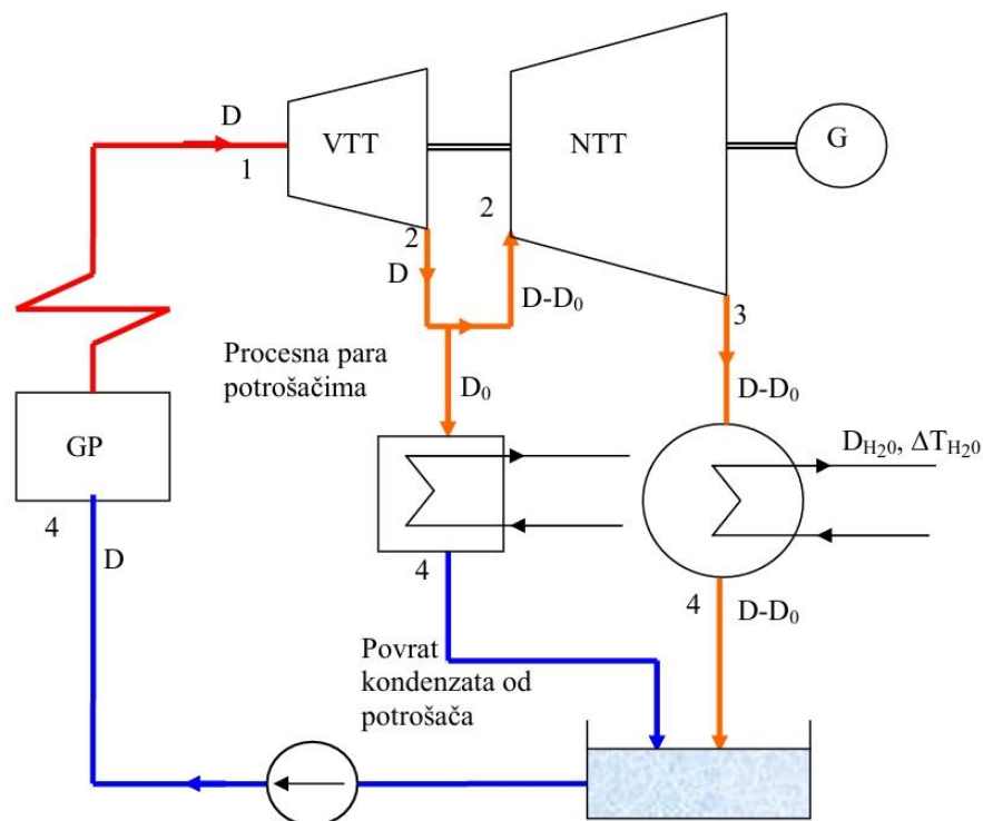
Slika 6: Shema parne turbine s reguliranim oduzimanjem pare [8].
