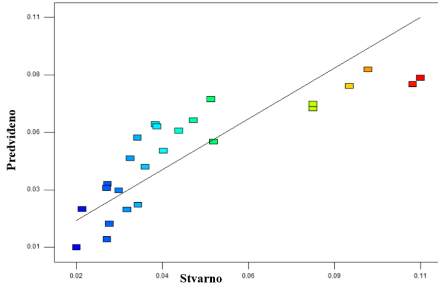
Slika 15. Usporedba eksperimentalnih i modelom predviđenih vrijednosti odziva za UV-C/H 2 O 2 proces.
