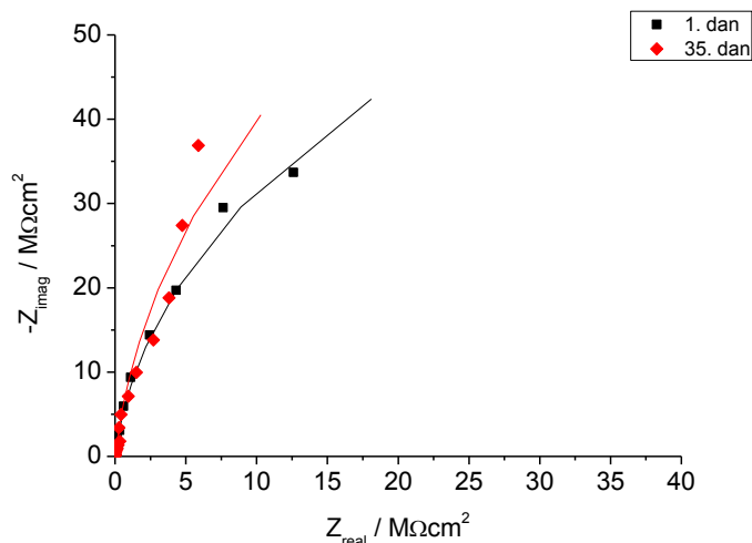
Slika 4.38. Nyquistov prikaz impedancijskih krivulja za sustav S5 (simboli –eksperimentalno dobiveni podaci, linije- podaci dobiveni modeliranjem)
