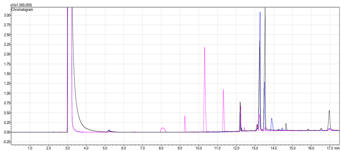
Slika 31. Kromatogram biodizela; FBE 1 – crno; FBE 2 – rozo; FBE 3 – plavo
