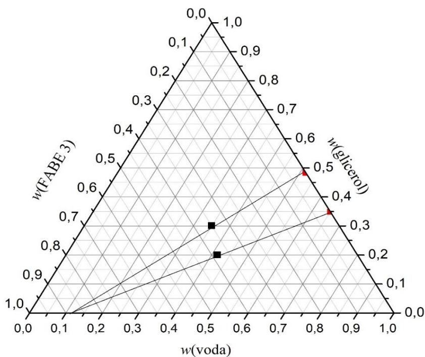
Slika 24. Fazni dijagram sustava voda – glicerol – FABE 3 (pročišćeni). Crne točke – početni pseudotrokomponentni sastavi; crvene točke na stranici trokuta – ravnotežni sastavi; crne linije – vezne linije
