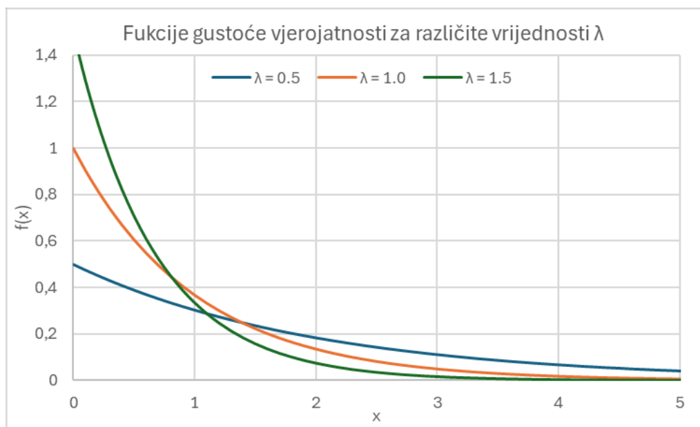
Slika 11. Funkcija f za eksponencijalnu slučajnu varijablu
