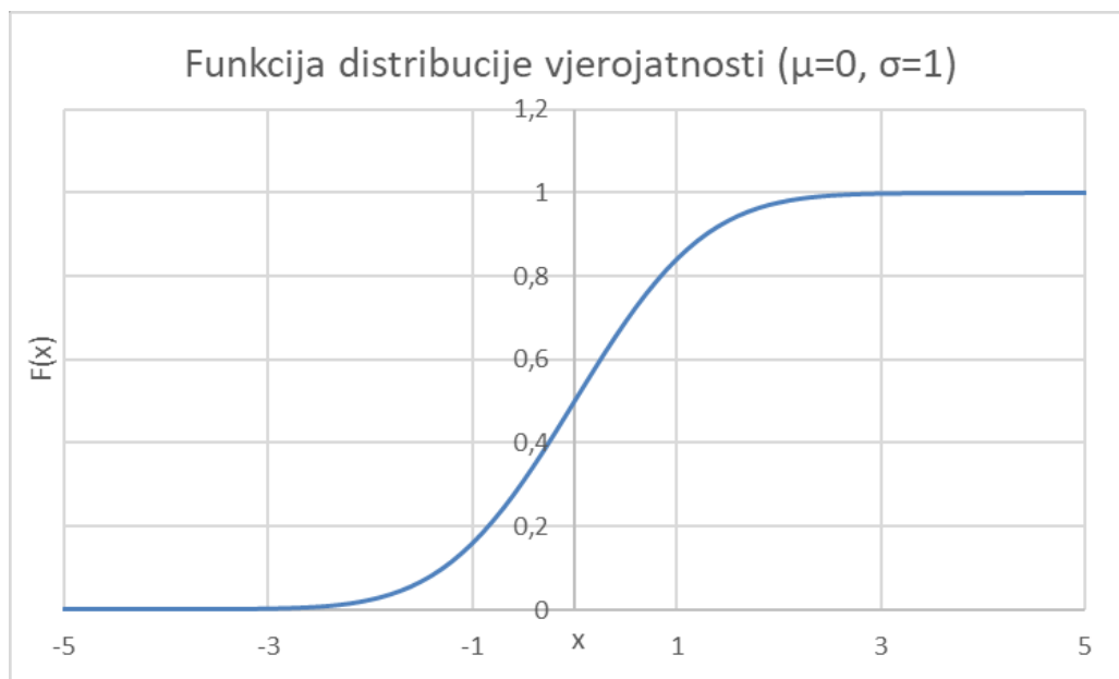
Slika 7. Funkcija distribucije vjerojatnosti standardne normalne slučajne varijable
