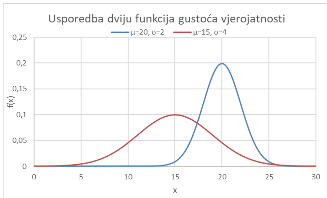
Slika 5. Usporedba dviju funkcija gustoća vjerojatnosti
