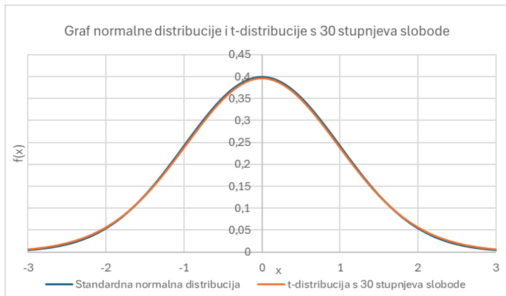
Slika 24. Graf normalne distribucije i t-distribucije s 30 stupnjeva slobode
