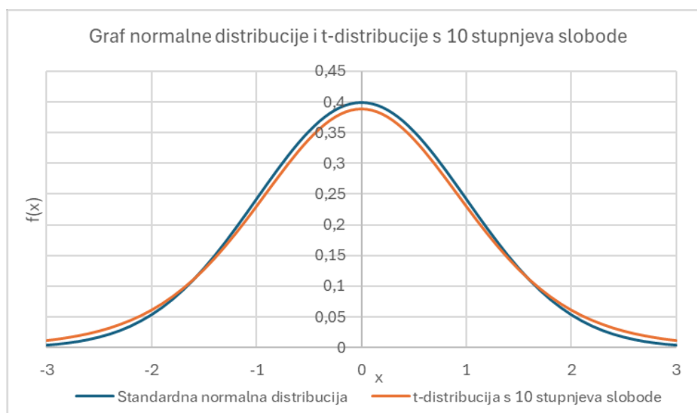
Slika 22. Graf normalne distribucije i t-distribucije s 10 stupnjevima slobode
