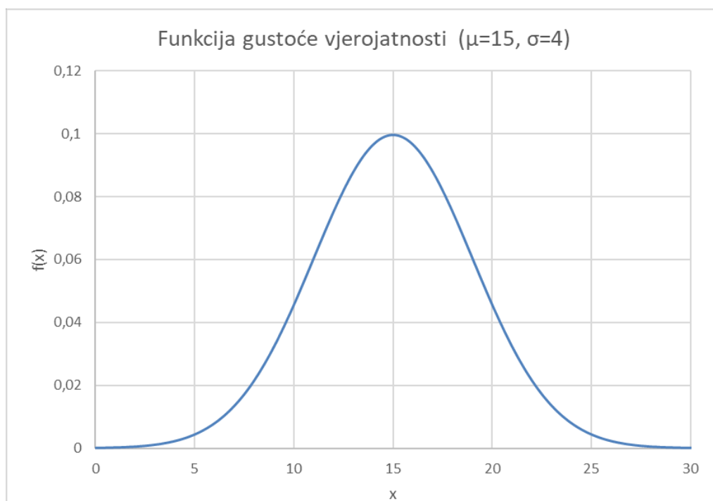
Slika 3. Funkcija gustoće vjerojatnosti ( \mu=15 i \sigma=4 )
