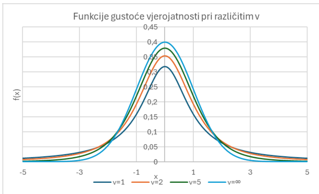
Slika 19. Funkcija f za Studentovu t-distribuciju
