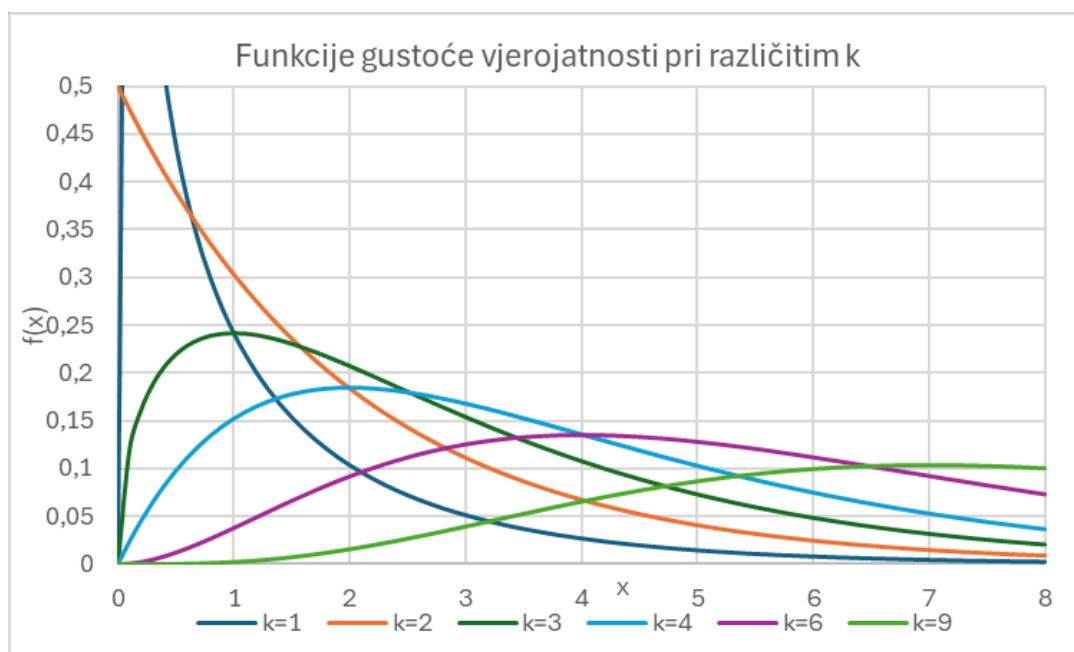
Slika 25. Funkcija f za hi-kvadrat distribuciju
