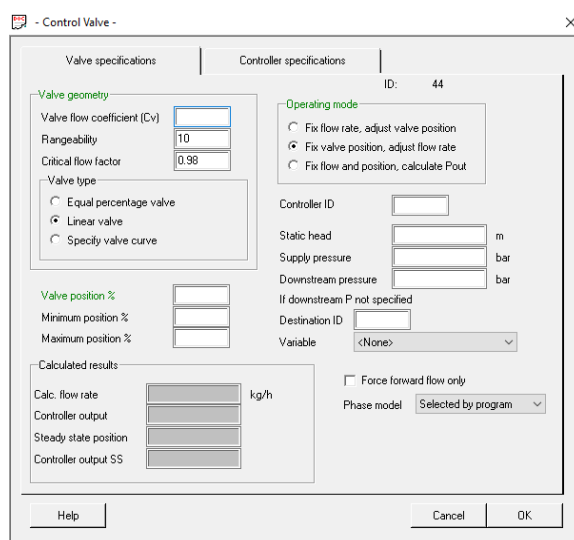
Slika 3.12. Definiranje regulacijskog ventila
