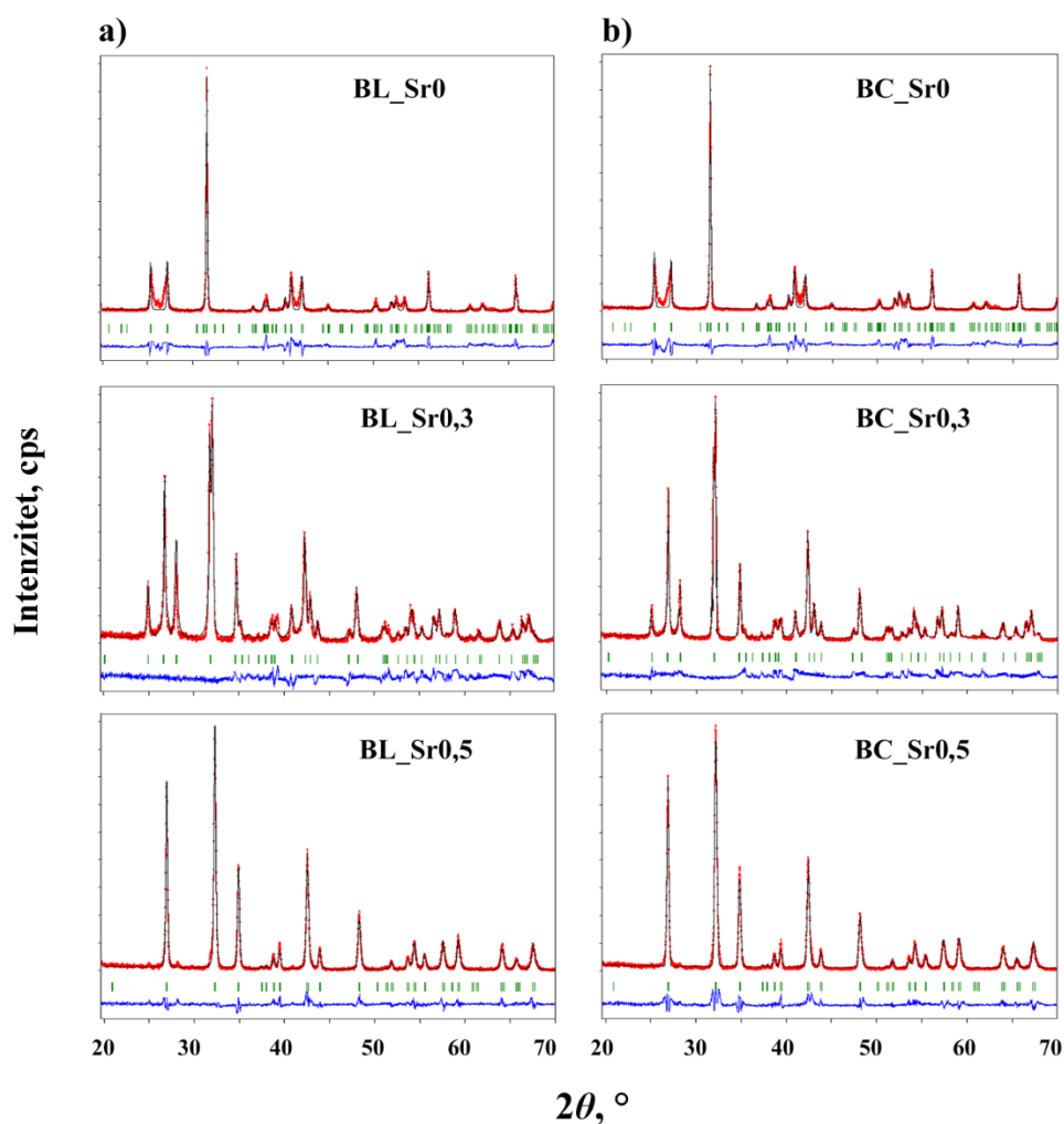
Slika 29. Rezultati Rietveldove metode utočnjavanja za BSMO-uzorke pripremljene (a) limunskim i (b) koprecipitacijskim postupkom sinteze. Eksperimentalni podaci prikazani su crvenim točkama, izračunati model crnom linijom, a odstupanja eksperimentalnih podataka od modela prikazana su plavom linijom ispod difraktograma. Zelenim crtama prikazane su Braggove pozicije za svaku od faza.
