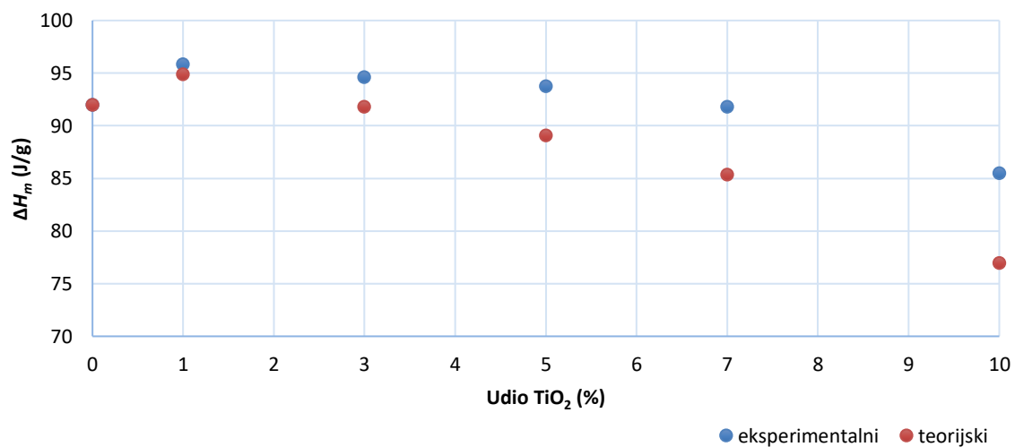
Slika 20. Promjena entalpije taljenja u nanokompozitima PHBV/ \text{TiO}_2
