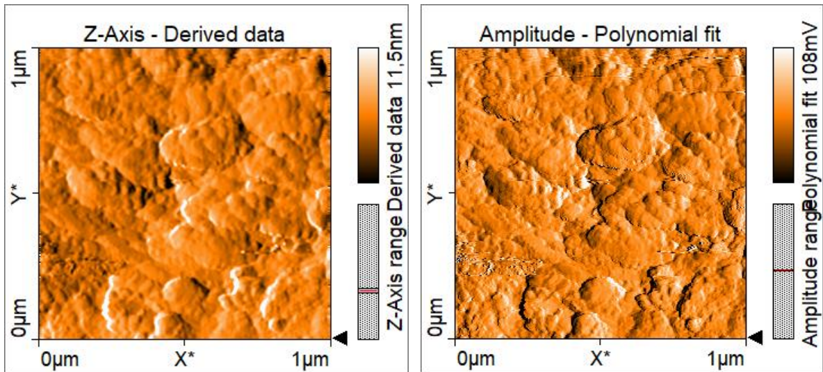
Slika 20. AFM mikrografije početnog sloja dobivenog metodom ablacije iskrom pri protoku 3 L/min, dimenzije 1 x 1 μm 2
