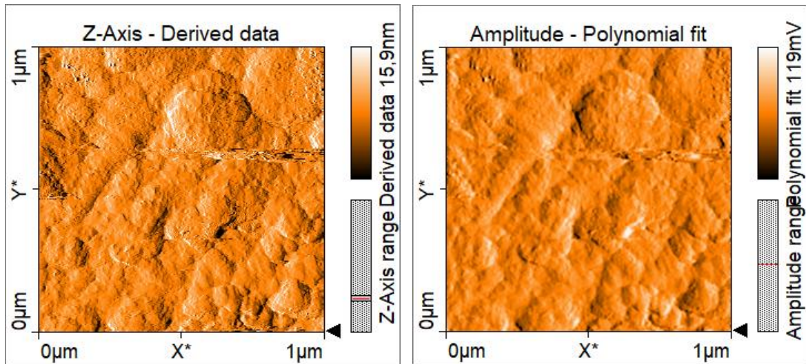
Slika 21. AFM mikrografije početnog sloja dobivenog metodom ablacije iskrom pri protoku 5 L/min, dimenzije 1 x 1 μm 2
