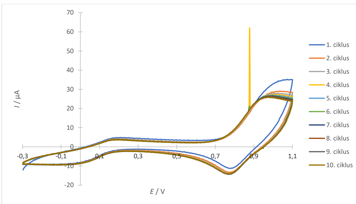
Slika 41. Odziv GC elektrode oslojene s PB, laktat oksidazom i kitozonom u osnovnom elektrolitu (0,1 M KCl). Snimano u troelektrodnoj elektrokemijskoj ćeliji uz uporabu Pt žice kao pomoćne elektrode i zasićene Ag/AgCl referentne elektrode uz brzinu promjene potencijala (engl. scan rate ) od 50 mV/s unutar potencijala od -0,3 V do 1,1 V.
