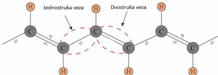
Slika 2.4. Prikaz konjugirane dvostruke veze elektrovođljivih polimera [9]
