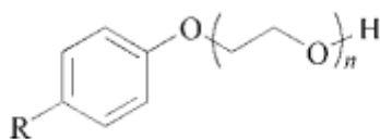
Slika 10. Alkil fenol etoksilat ( R=C_{8-12} , n=5-10 )
