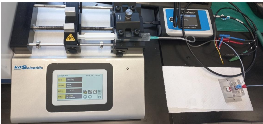
Slika 11. Pumpa za špricu ( KD Scientific, Legato 200 Series ) i potencijostat ( PalmSens4 )
