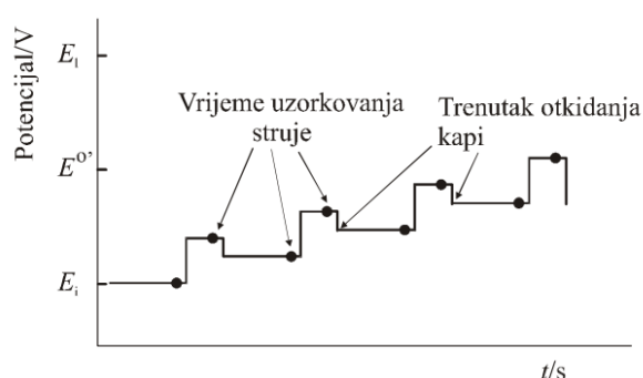
Slika 5. Signal pobude (a) i odziva (b) za diferencijalnu pulsnu voltametriju [11].
