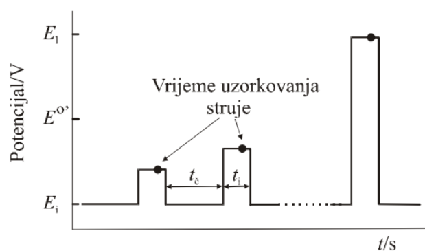
Slika 4. Signal pobude za pulsnu voltametriju [11].
