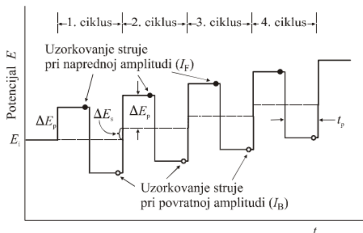
Slika 6. Prikaz signala pobude i vremena uzorkovanja struje u pravokutnovalnoj voltametrij [11].
