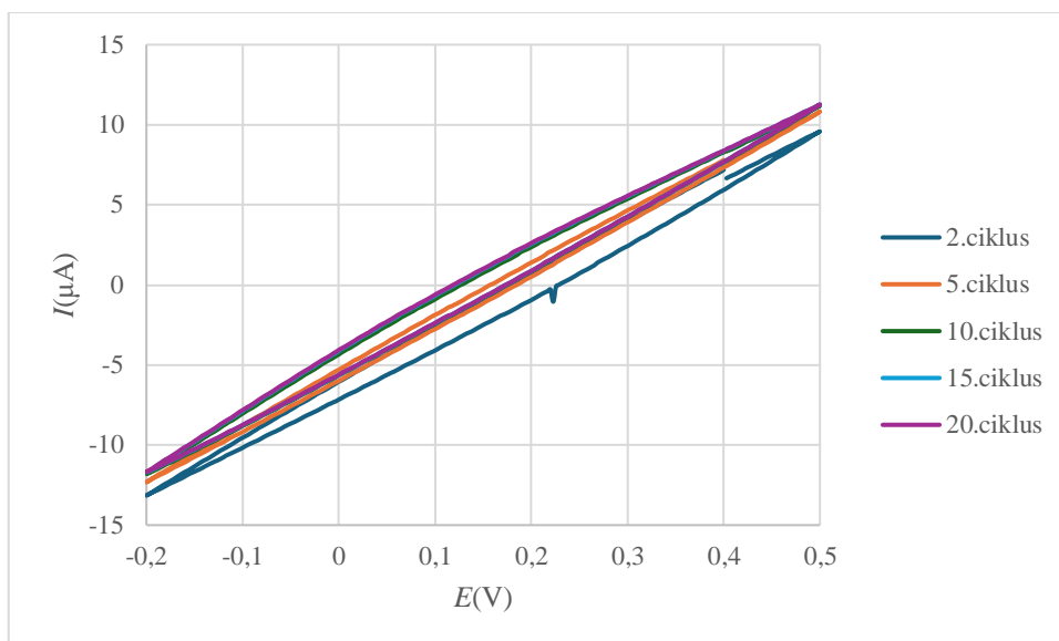
Slika 52: Graf aktivacije sloja berlinskog modrila na inkjet ispisanjoj elektrodi u \text{KCl} (2; 5; 10; 15. i 20. ciklus) (60 min depozicije)
