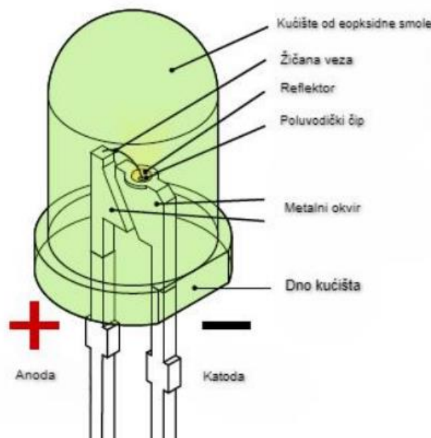
Slika 5.3. LED dioda
