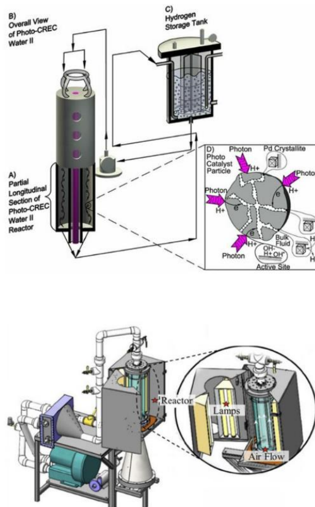
Slika 4.4. Foto-CREC-reaktor
