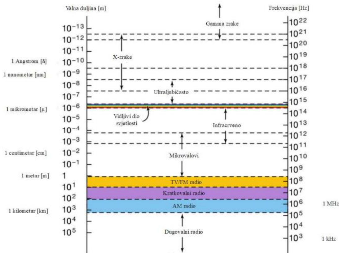
Slika 3.3. Elektromagnetski spektar
