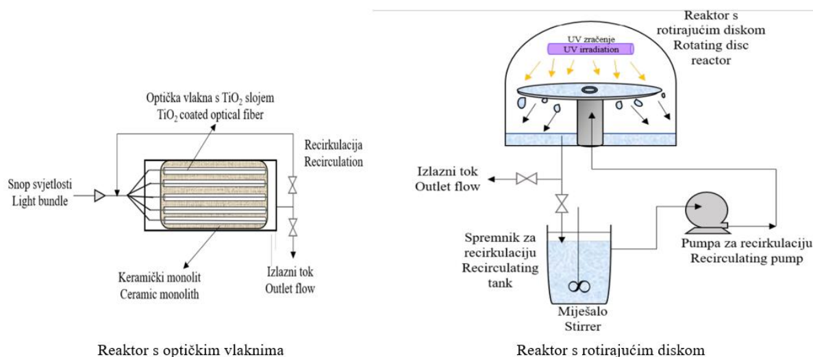
Slika 4.6. Reaktor s optičkim vlaknima i rotirajućim diskom
