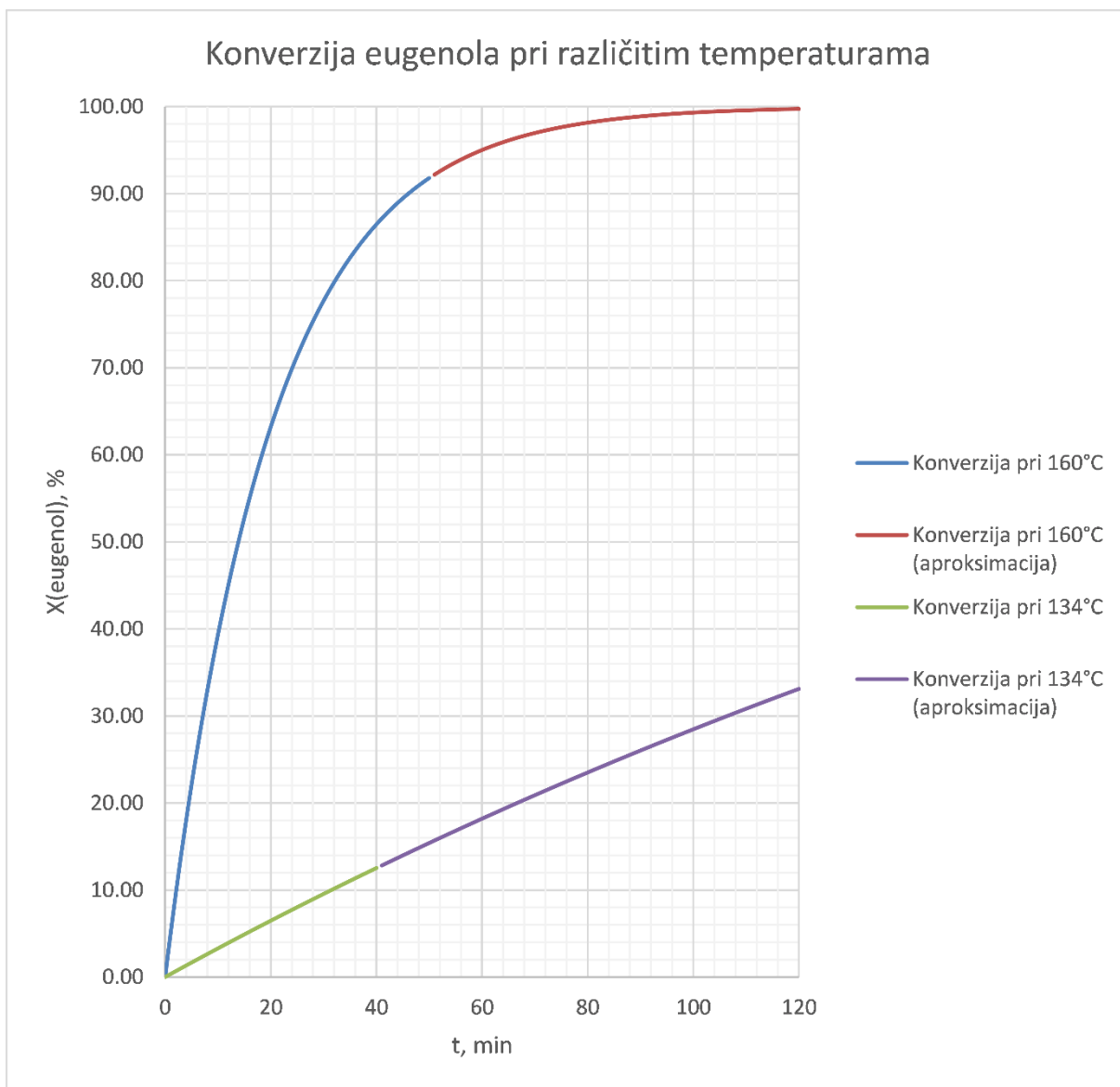
Slika 3.11: Grafički prikaz literaturne [32] i aproksimirane ovisnosti konverzije 2-metoksi-4-(prop-2-en-1-il)fenola [X(eugenol)] o vremenu (t) pri različitim temperaturama
