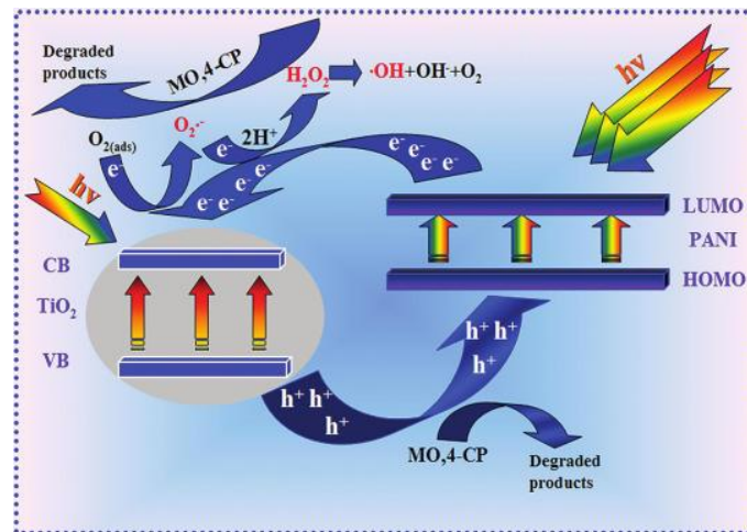
Slika 2. Sinergijski efekt PANI/ \text{TiO}_2 gdje je prikazano kako i vidljiv dio Sunčevog zračenja doprinosi fotokatalitičkoj razgradnji putem \text{TiO}_2 .
