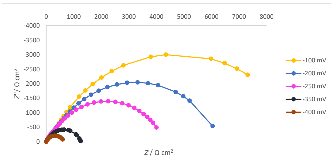
Slika 4.6. Nyquistov prikaz impedancijskih spektara Zr elektrode u 1 mol dm -3 otopini NaOH pri naznačenim prenaponima za reakciju razvijanja vodika
