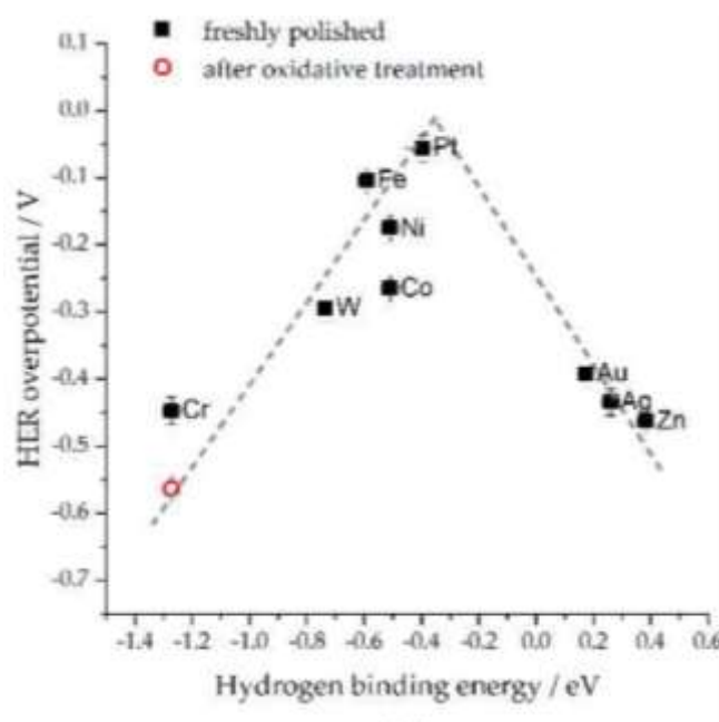
Slika 2.4. Vulkanski prikaz reakcija razvijanja vodika u alkalnom mediju 1 \text{ mol dm}^{-3} \text{ KOH} 20
