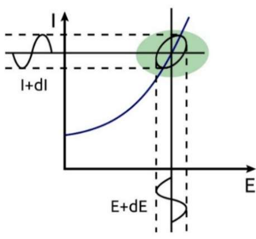
Slika 3.8. Lissajousov dijagram 47
