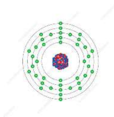
Slika 2.6. a) Čisti cirkonij 25 b) Prikaz cirkonijeve jezgre i elektronskog omotača 26
