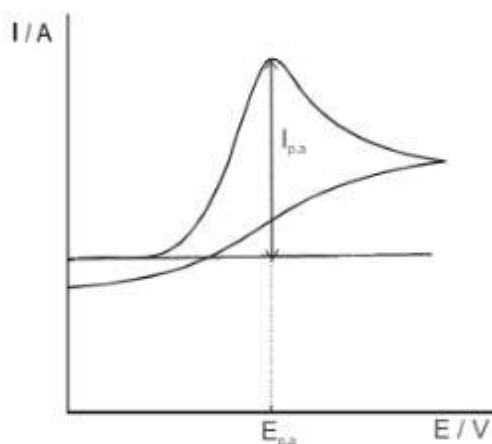
Slika 3.6. Ciklički voltamogram ireverzibilnog procesa 15
