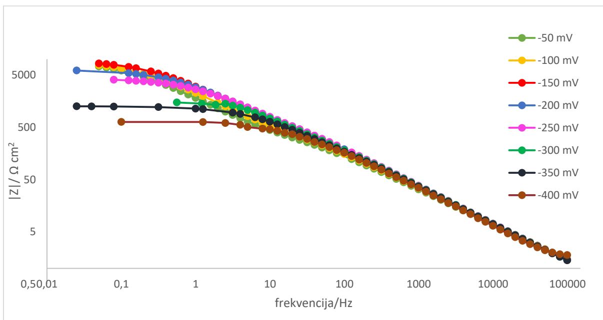
Slika 4.7. Bodeov prikaz impedancijskih spektara Zr elektrode u 1 mol dm -3 otopini NaOH pri naznačenim prenaponima za reakciju razvijanja vodika
