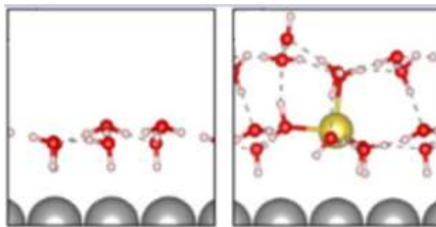
Slika 2.5. Model za \text{H}_2\text{O} kao izvor protona; žutim je označen kation \text{Na}^+ i njegov točan položaj na elektrokemijskoj granici
