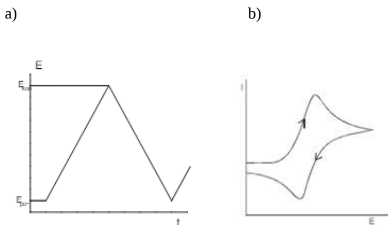
Slika 3.4. Signal a) pobude i b) odziva u cikličkoj voltametrij 15
