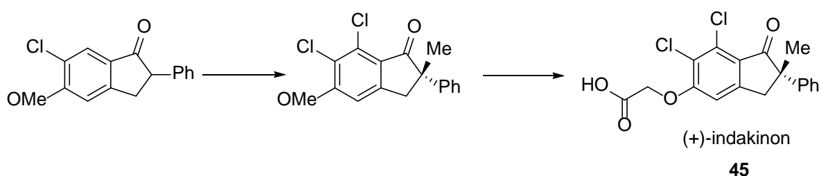
Shema 26. Sinteza urikozurika (+)-indakrinona
