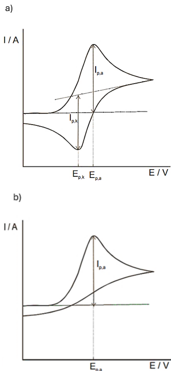
Slika 2.18. Ciklički voltamogram a) reverzibilni elektroodni proces, b) ireverzibilni elektroodni proces [60].
