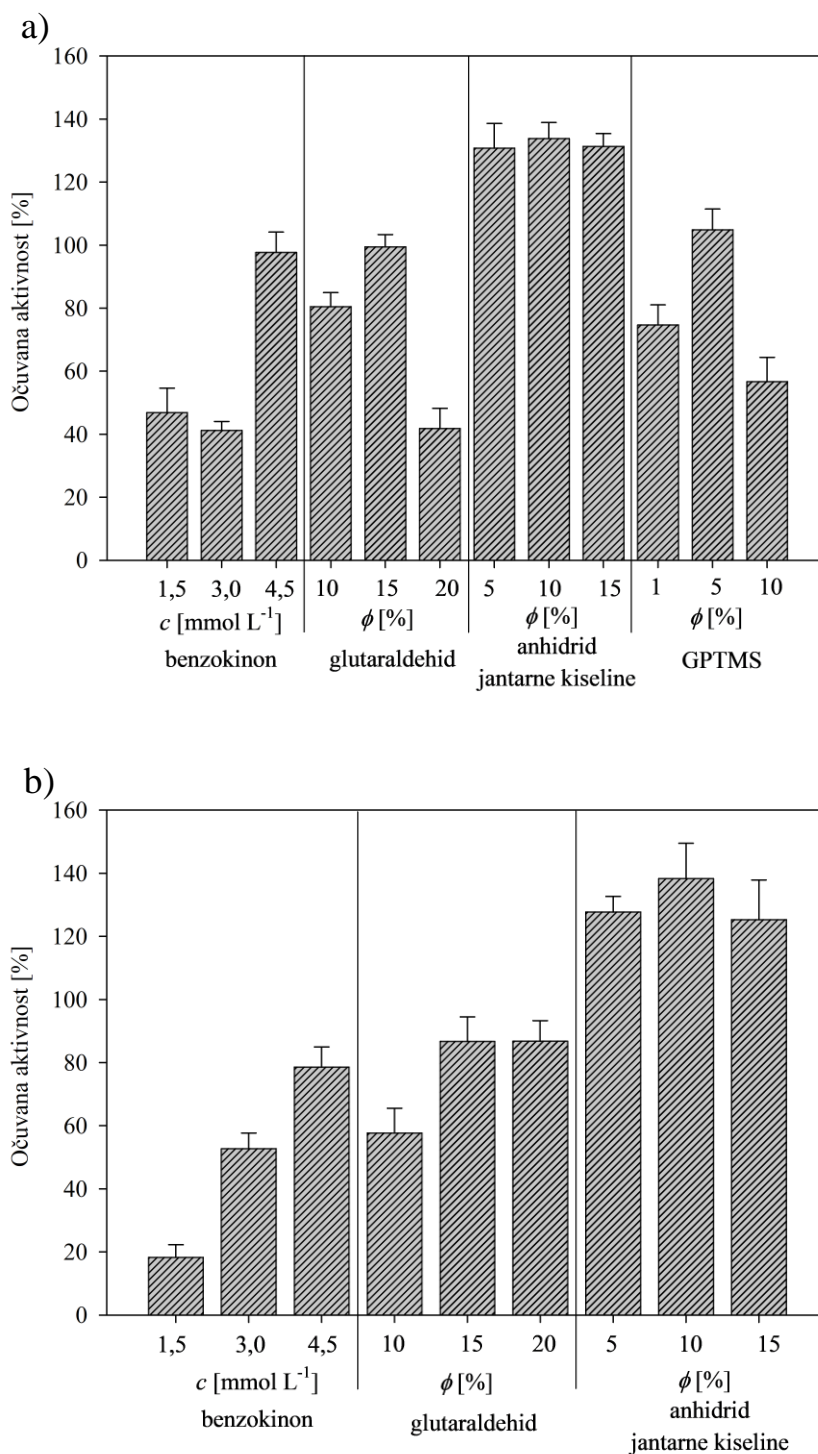
Slika 26. Utjecaj različitih koncentracija aktivacijskih agensa vezanih na APTES/GPTMS (a) i APTMS (b) na procesni pokazatelj očuvane aktivnosti (fosfatni pufer 0,1 mmol L -1 , pH 6, 25 °C).
