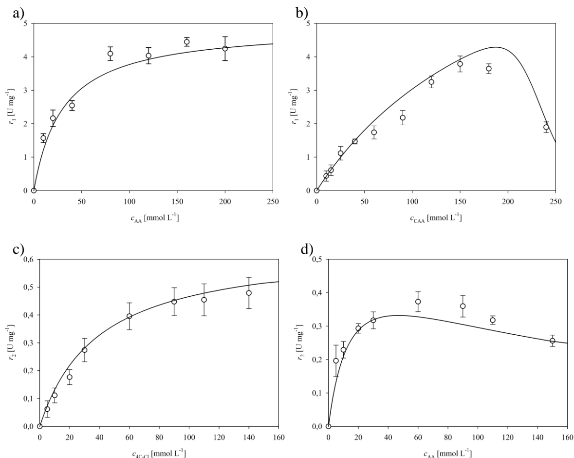
Slika 31. Kinetika DERA 024 imobiliziranog na MCF-b/APTMS/10 % anhidrid jantarne kiseline u reakciji prve (a, b) i druge (c, d) aldolne adicije. Prikazan je utjecaj različitih koncentracija: a -acetaldehida ( c_{CAA} = 150 \text{ mmol L}^{-1} ), b -kloroacetaldehida ( c_{AA} = 150 \text{ mmol L}^{-1} ), c -acetaldehida ( c_{4C-Cl} = 100 \text{ mmol L}^{-1} ) i d -4-kloro-3-hidroksibutanala ( c_{AA} = 50 \text{ mmol L}^{-1} ) na početnu brzinu reakcije (fosfatni pufer 0.1 \text{ mol L}^{-1} , pH 6, 25 \text{ }^\circ\text{C} , \gamma_{\text{DERA}^{024}} = 1 \text{ mg mL}^{-1} ).
