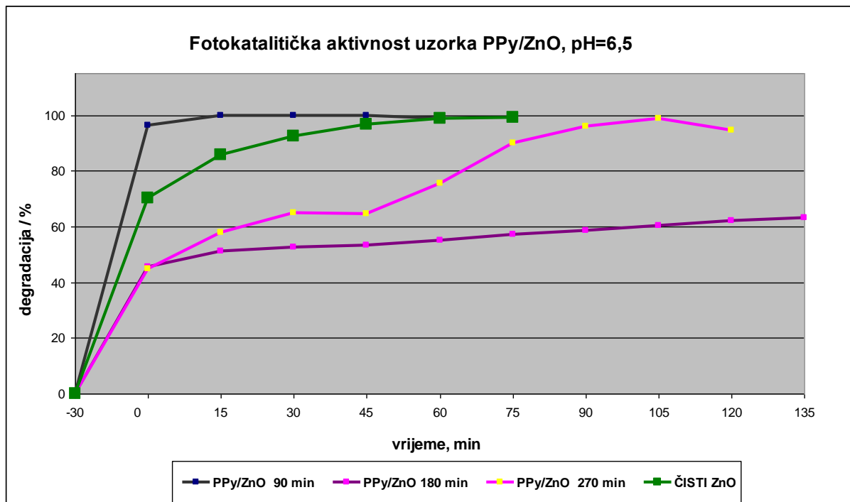
Slika 18. Stupanj degradacije bojila Reactive Red 45 na UV svjetlu pri pH=6,5 za ispitivane uzorke PPy/ZnO kompozita
