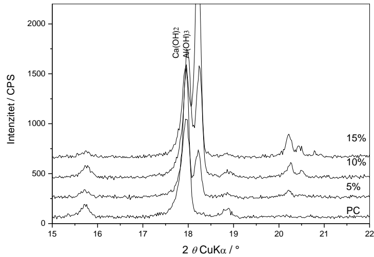
Slika 4-19. Detalj difraktograma sa slike 4-18. Vidljiv je sve veći difrakcijski maksimum aluminijeva hidroksida koji je djelomično preklopljen s difrakcijskim maksimumom \text{Ca(OH)}_2 . Uzorci sadrže 0, 5, 10 i 15% aluminijeva hidroksida.
