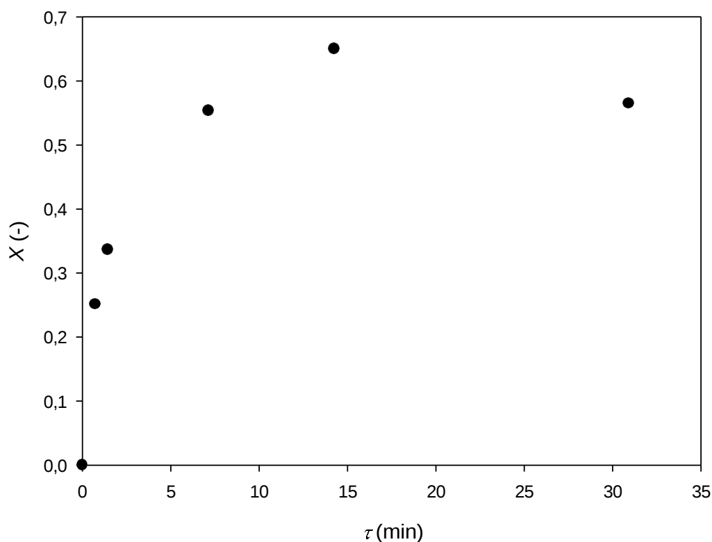
Slika 4.7 Utjecaj vremena zadržavanja na konverziju za reakciju polimerizacije apigenina u mikroreaktoru
