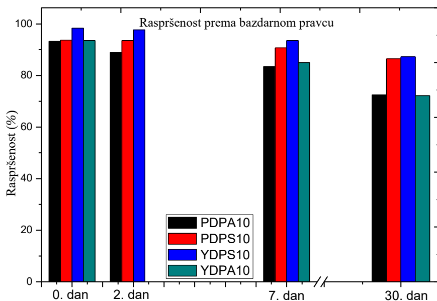
Slika 4.2.18. Raspršenost nanofluida nakon gravitacijske sedimentacije (prema baždarnom pravcu)
