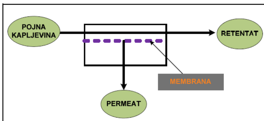
Slika 7. Membransko razdvajanje ulazne struje na struju retentata i permeata 7
