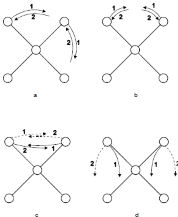
Slika 7: Prikaz vibracija deformacija višeatomne molekule. Strelice označene punom crtom označavaju gibanje jezgara iznad, a crtanim ispod ravnine papira
