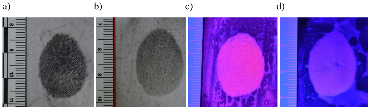
Slika 28. Otisci prsta izazivani prahovima a) instant crni, b) supranano crni, c) fluorescirajući magnetični crveni i d) supranano fluorescirajući crveni magnetični na prozirnoj plastici 10 dana nakon nanošenja.
