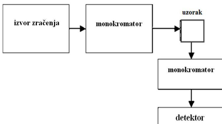
Slika 5. Shema fluorimetra [6]
