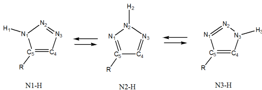
Slika 15. Tautomeri 1,2,3-triazola
