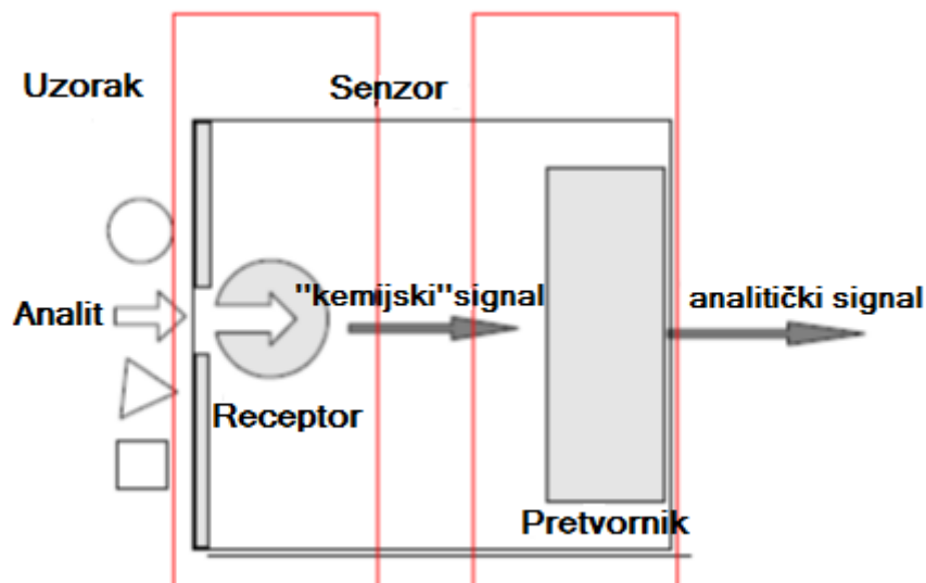
Slika 2.1. Kemijski senzor
