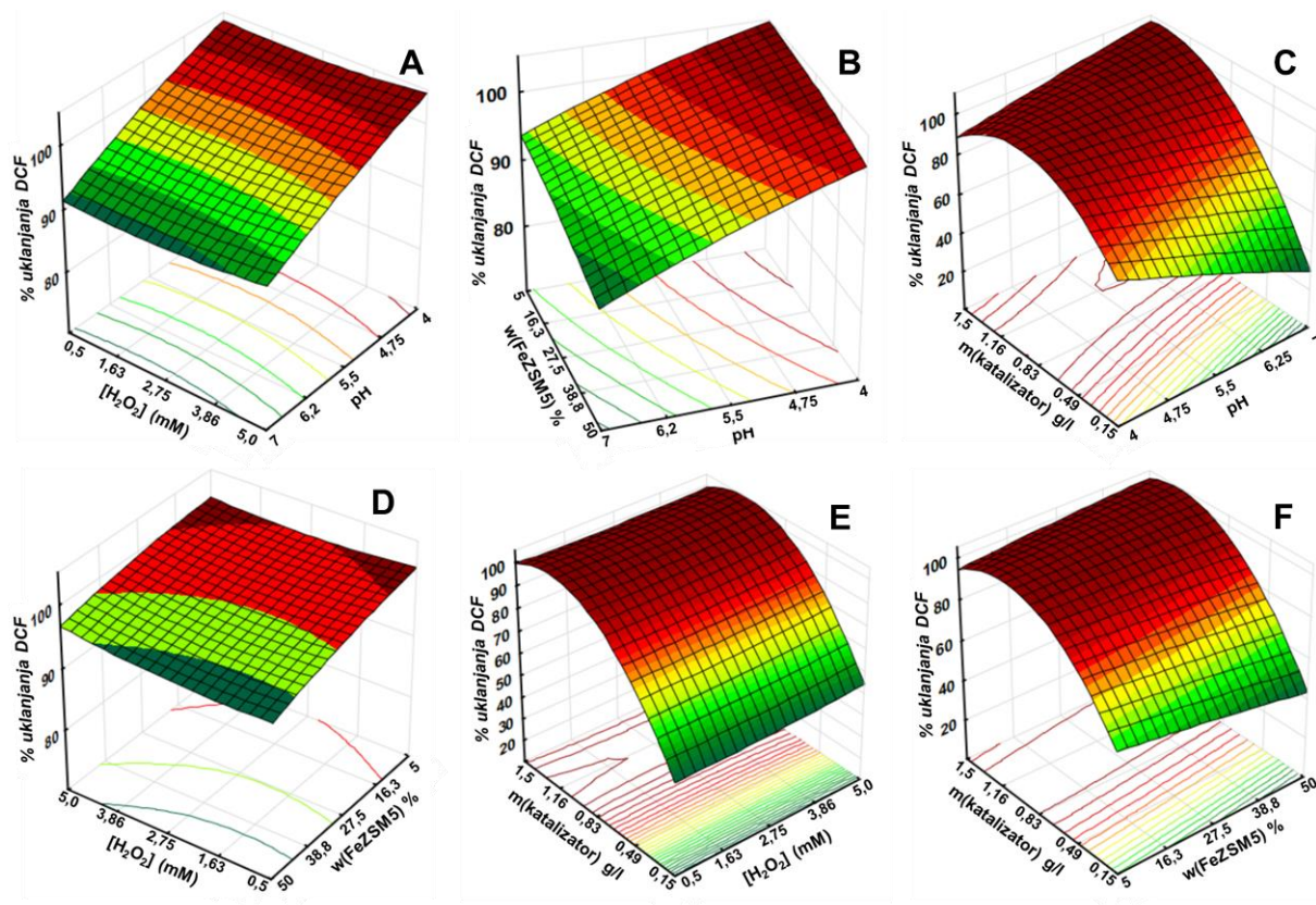
Slika 19. 3D dijagrami međuutjecaja procesnih parametara Solar/TiO 2 -FeZSM5 procesa na učinkovitost uklanjanja DCF-a; A) pH i [H 2 O 2 ], B) pH i w(FeZSM5), C) pH i γ(katalizator), D) [H 2 O 2 ] i w(FeZSM5), E) [H 2 O 2 ] i γ(katalizator), F) w(FeZSM5) i γ(katalizator)
