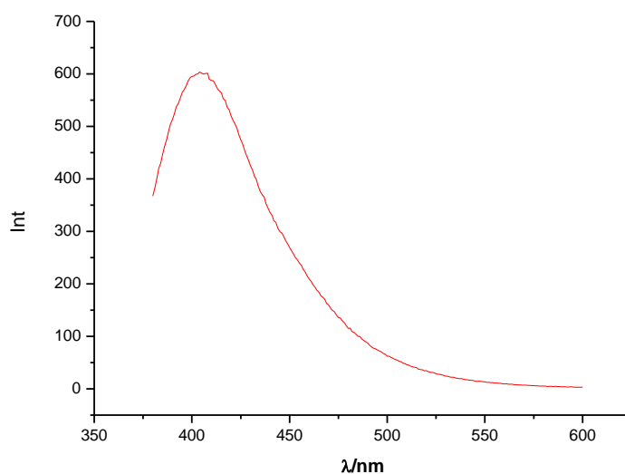
Slika 8. Emisijski spektar spoja 2 ( c = 1 \times 10^{-8} \text{ mol dm}^{-3} )
