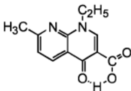
Slika 3. Nalidiksična kiselina [8]
