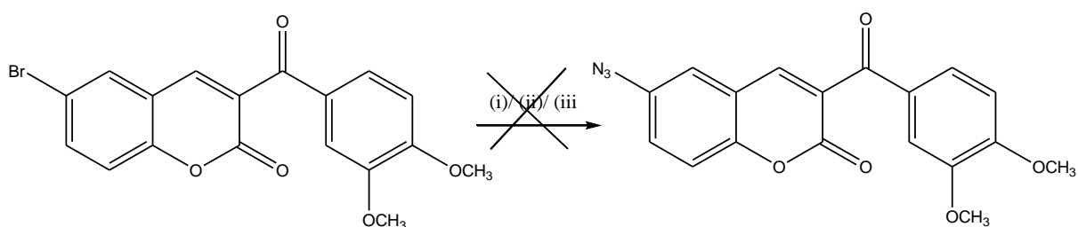
Shema 3. Reagensi i uvjeti: (i) \text{NaN}_3 , CuI, refluks, (ii) \text{NaN}_3 , DMF, refluks, (iii) CuI, natrijev askorbat, alkin, \text{NaN}_3
